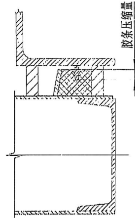
图 3 嵌压式
