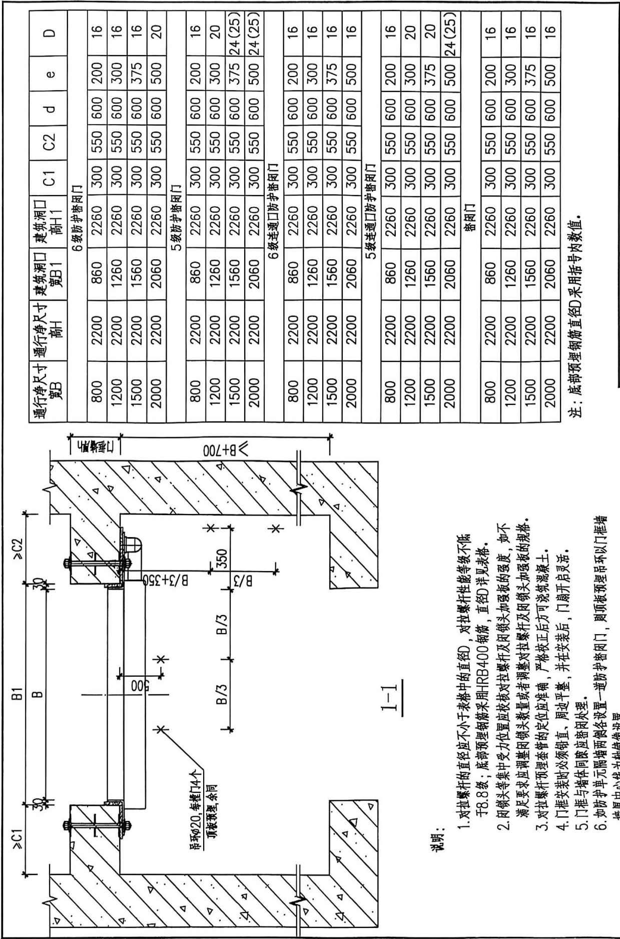
固定门槛单扇防护密闭门、密闭门(二) 连通口双向受力固定门槛单扇防护密闭门(二)
