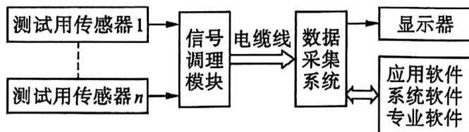
图C.2 抗力性能测试系统工作原理示意图
