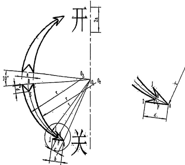
图 6 开关指示箭形标志尺寸示例
