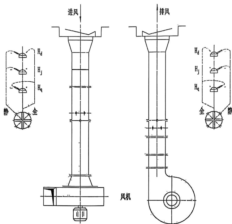
图 G.2 通风性能试验测试系统连接图
