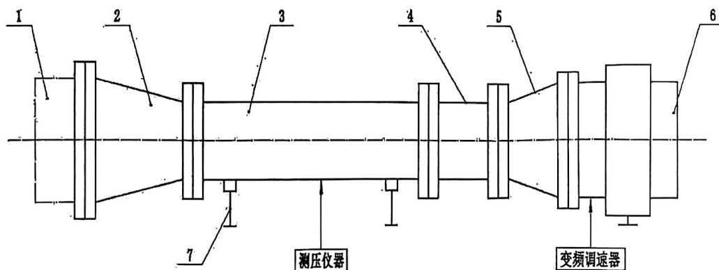
图 G. 1 通风性能试验装置示意图
