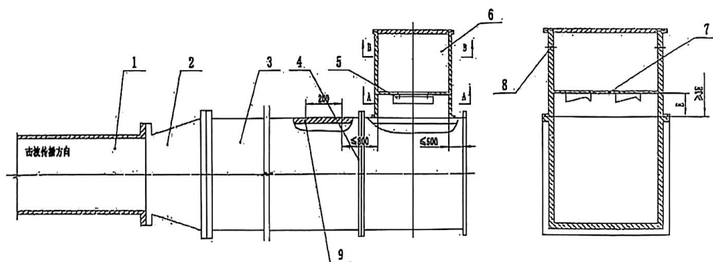
(a) 击波正向进入试验装置
