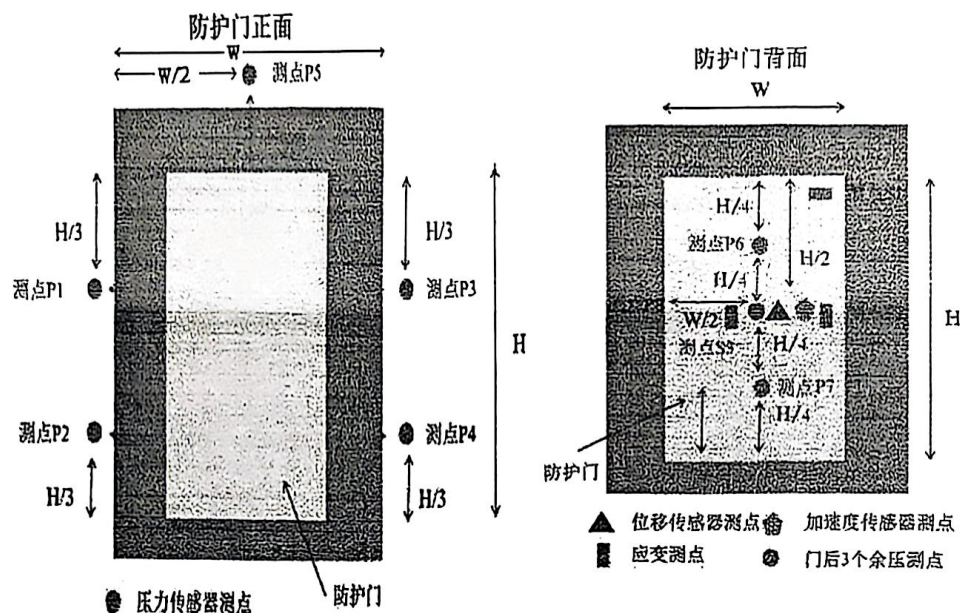
图A.4 传感器布点示意图
