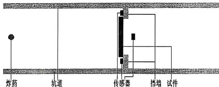
图 A. 3 试验装置示意图 (a-a)
